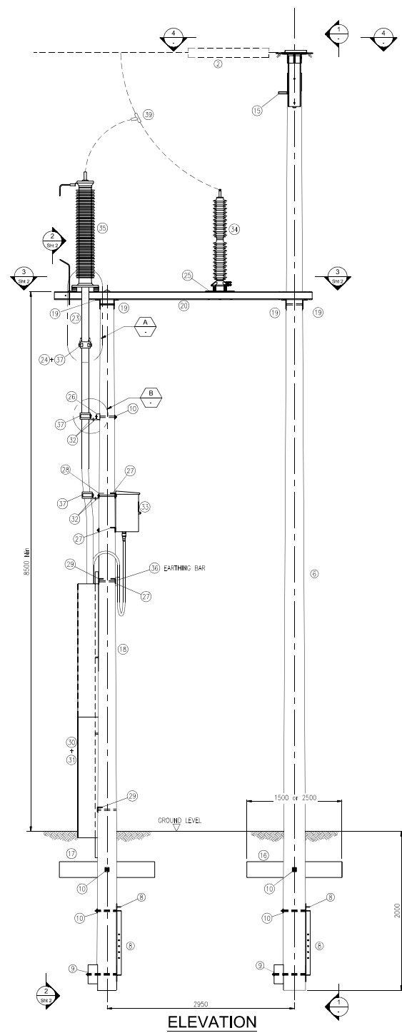
ELEVATION
